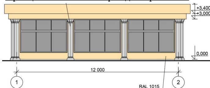
принципиальная схема фасадных решений:
