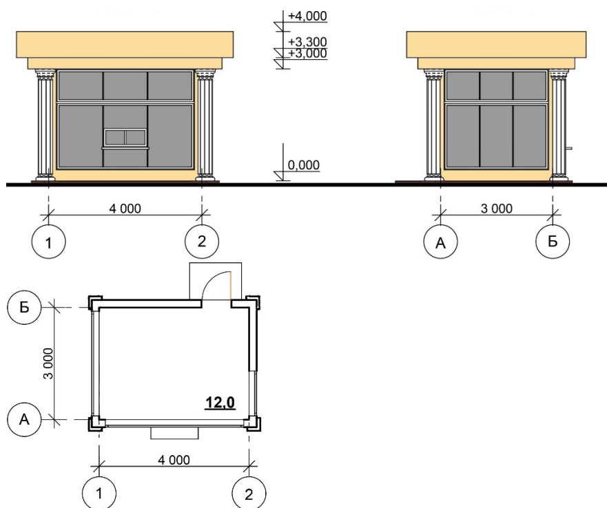
Рис. «Основные параметры места размещения нестационарного торгового объекта для киосков»
