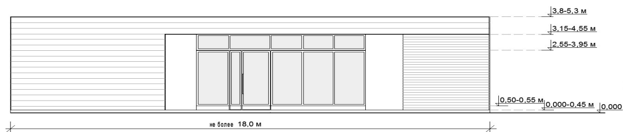
схема с максимальными размерами:
