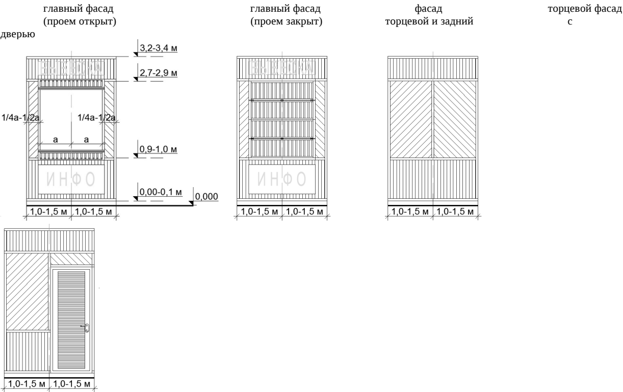
Рис. «Допустимые варианты габаритов элементов модулей жесткой палатки при планировании установки»
