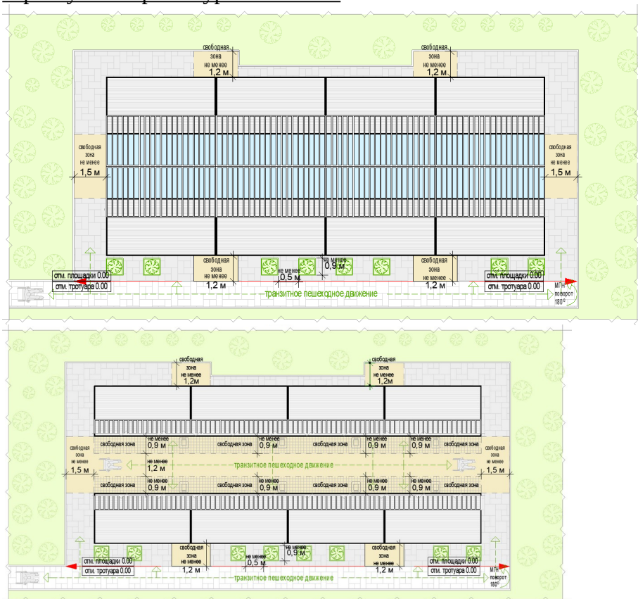
Схемы места размещения нестационарного торгового объекта при высоте входа в торговую галерею в уровне земли:
