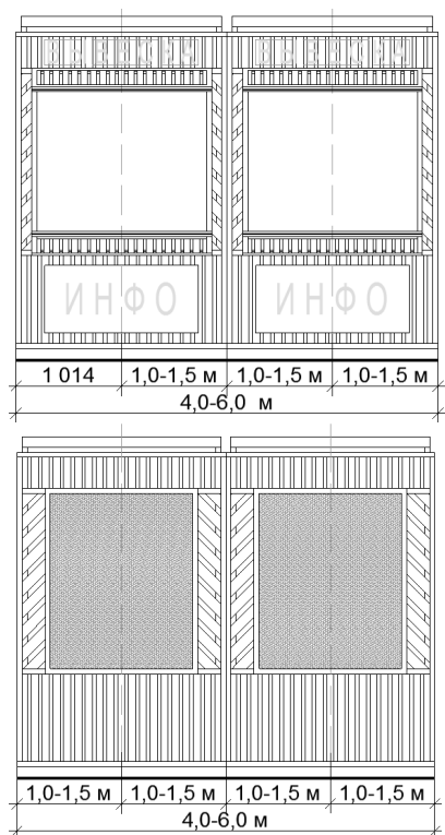
Рис. «Основные параметры места размещения нестационарного торгового объекта для палаток»
