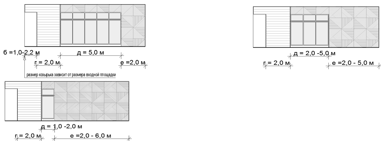
схема допустимого изменения баланса фасадных поверхностей (торцевой фасад):
